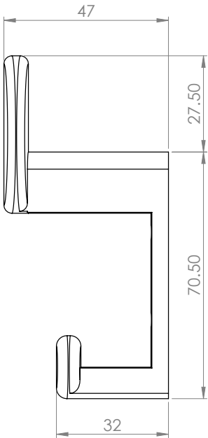
R.SIDE
